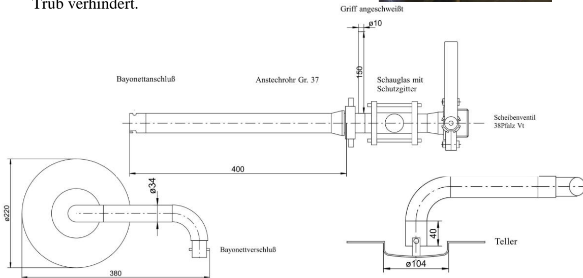
Abstichvorrichtung 2024-1 Stand 08.01.24
