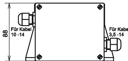
Ansicht auf Anschlusskasten
