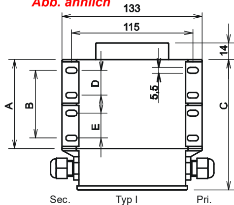
Abmessungen
